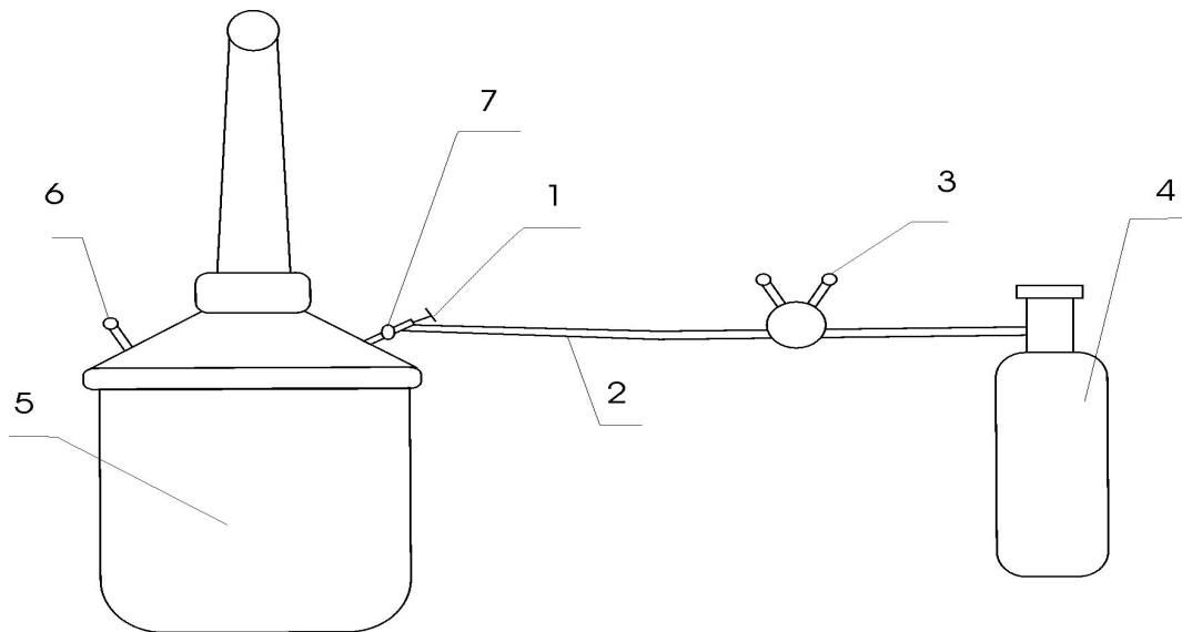
1、充气阀 2、氧气管道 3、氧气表 4、六氟化硫钢瓶 5、变压器
