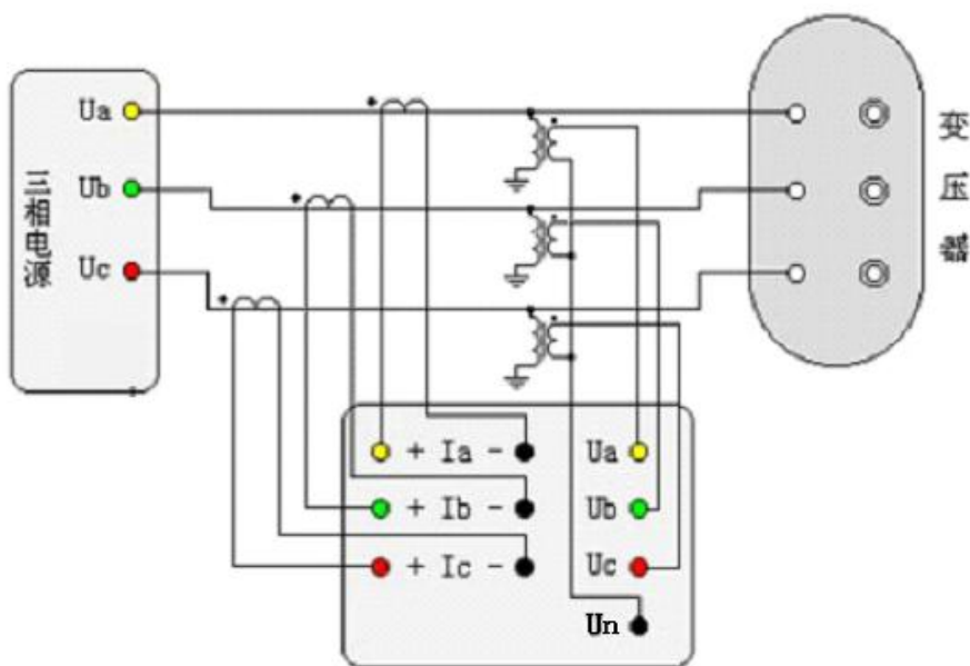
图二十八 三相空载损耗测试的直接接线示意图
