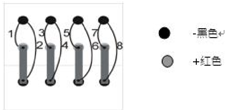
图 3. 2. 3-2 测试电池极柱和连接条的顺序
