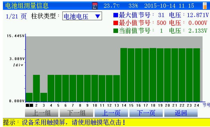
图 4.5.4-1 电池组柱状图界面
