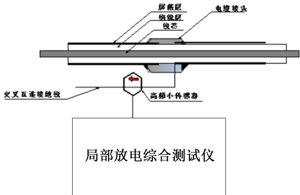
电缆接头局放在线现场连接示意图
