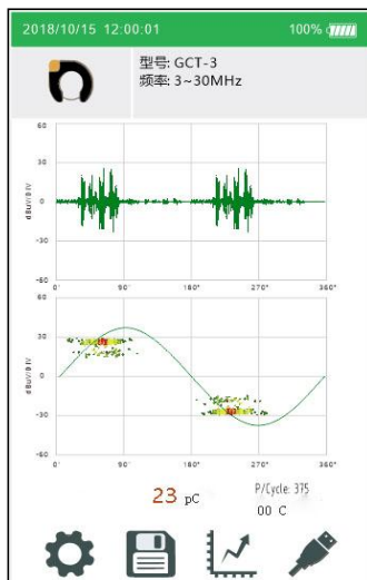
HFCT 测试界面
