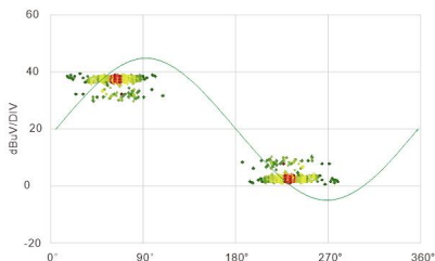
PRPD 图谱
