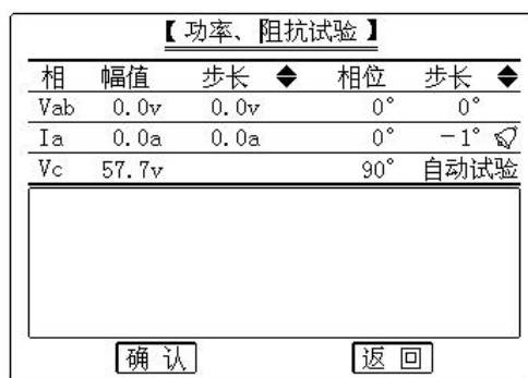
功率阻抗
