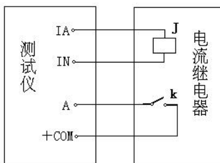
试验接线简图
