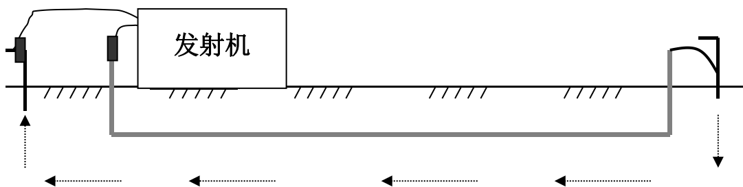
直连式测试法示意图
