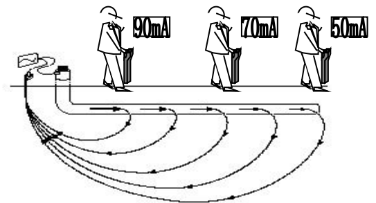
被测管线绝缘不良时探测示意图
