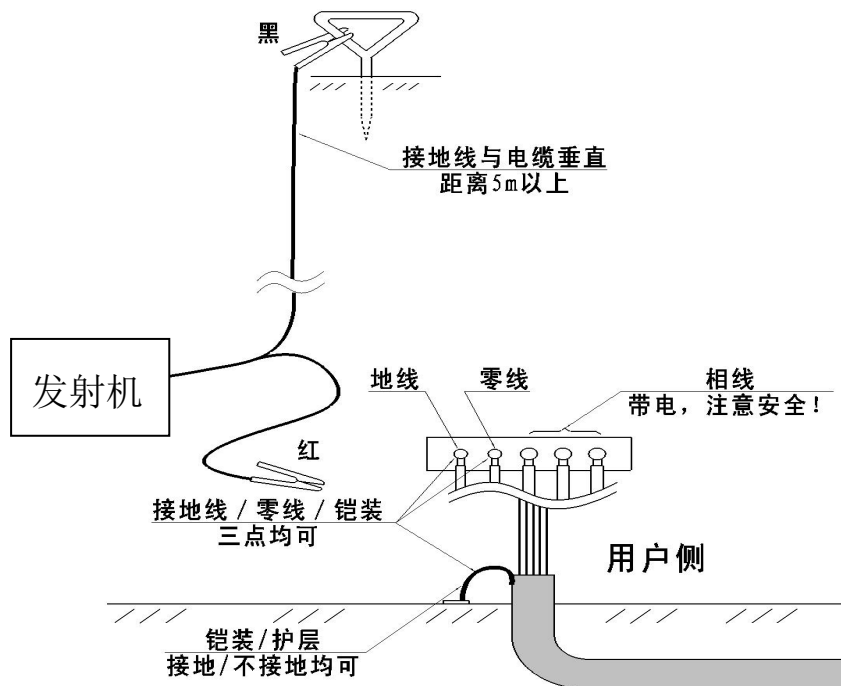
图 4.6 零线 / 地线 / 护层注入法
