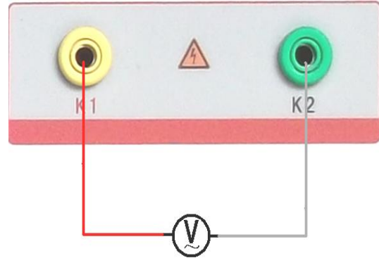
图 45，电压校准接线图
