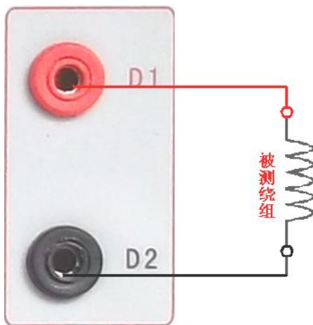
图 24，导线阻值清零接线图
