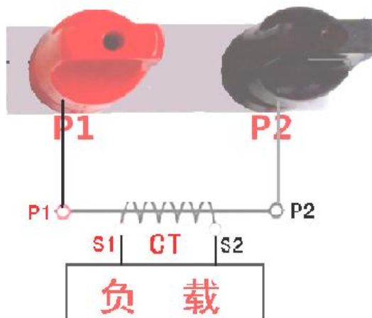
图 17、CT 一次通流接线图
