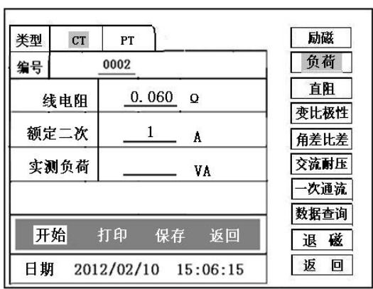
图 20, CT 二次负荷测试界面
