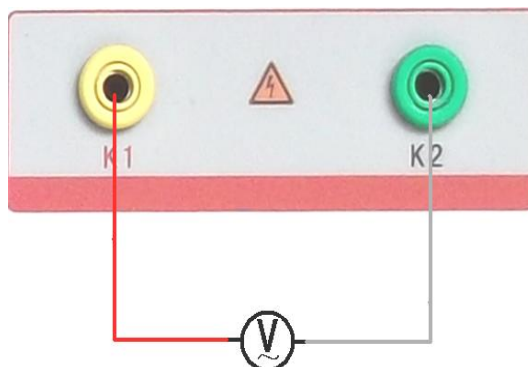
图 43，电压校准接线图
