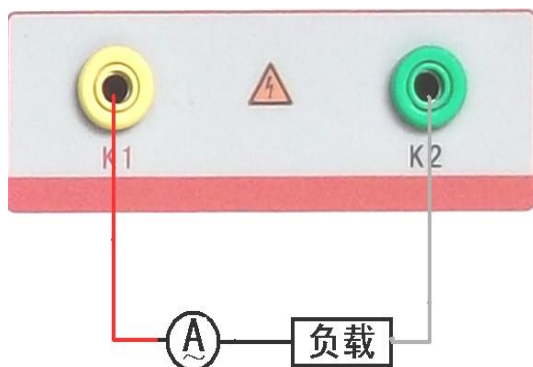
图 44，电流校准接线图
