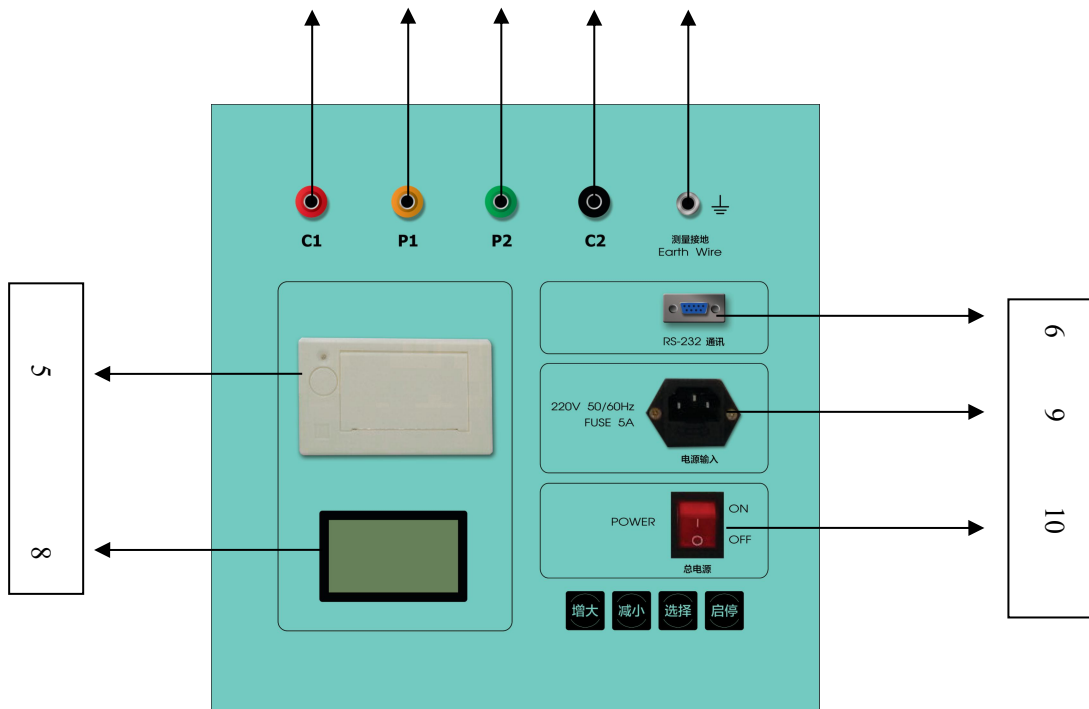
电源主机面板示意图
