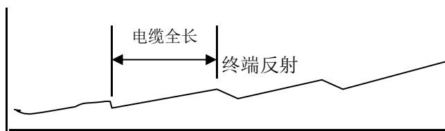
电缆故障点未被击穿时的测试波形
