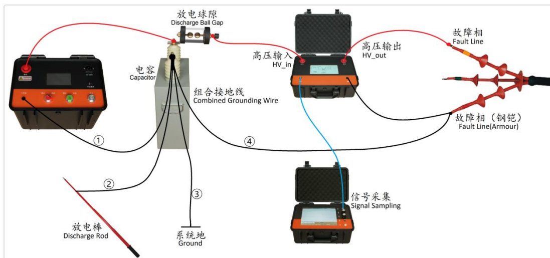
多次脉冲法连线示意图 The diagram of Multiple Pulse Method
