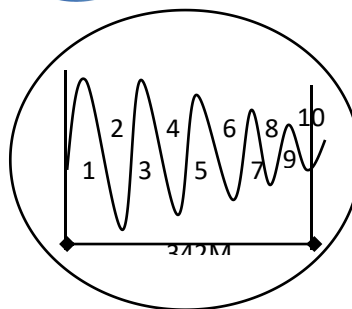
图 27 故障点在始端的波形放大
